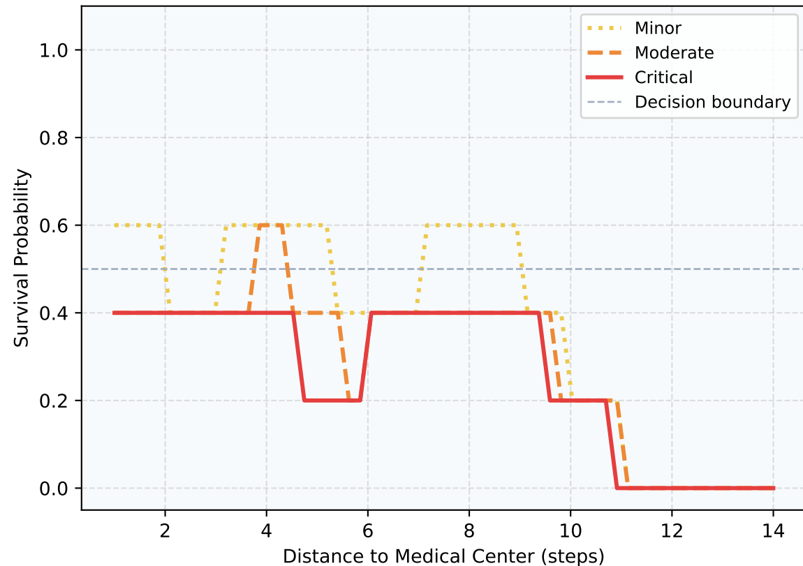
kNN (k=5)
